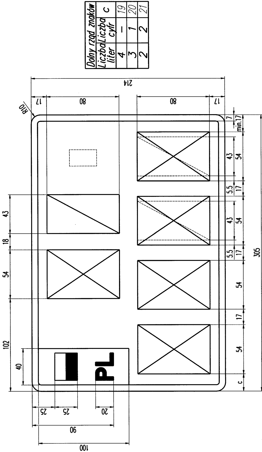
Rysunek 31. Tablica samochodowa indywidualna dwurzędowa
