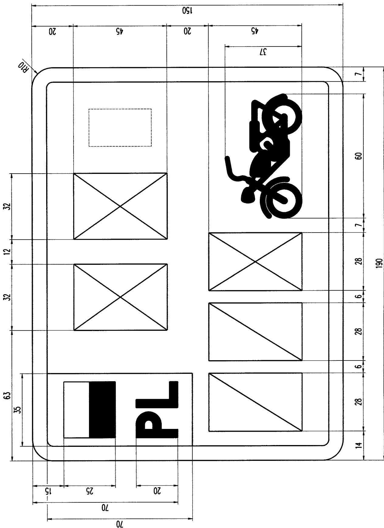
Rysunek 54. Tablica motocyklowa zabytkowa (2 litery, 2 cyfry, 1 litera)
