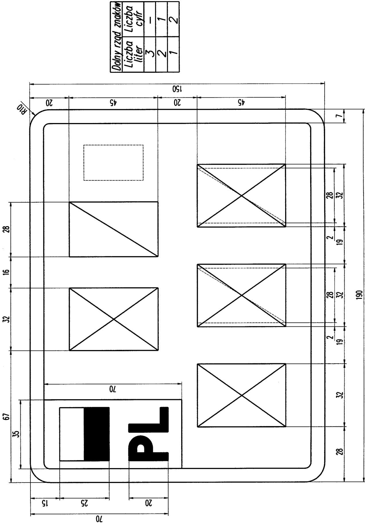
Rysunek 42. Tablica motocyklowa indywidualna
