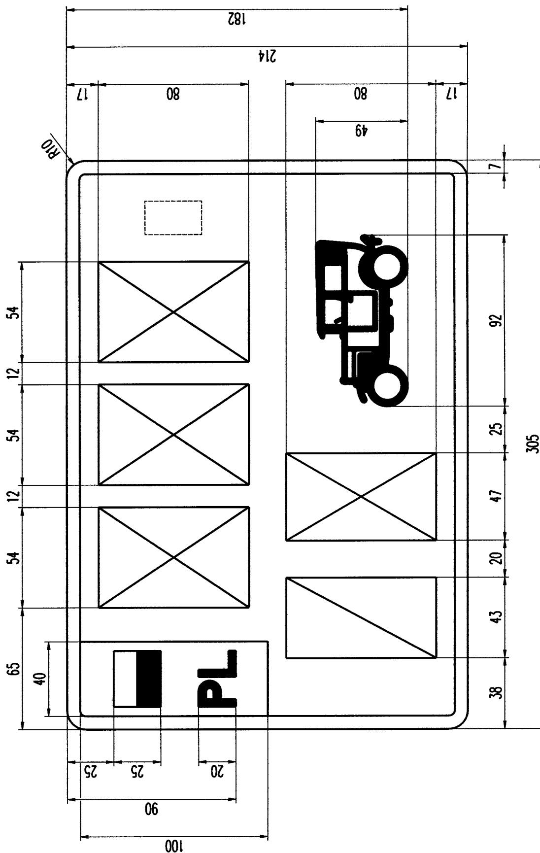
Rysunek 53. Tablica samochodowa zabytkowa dwurzędowa (3 litery, 1 cyfra, 1 litera)
