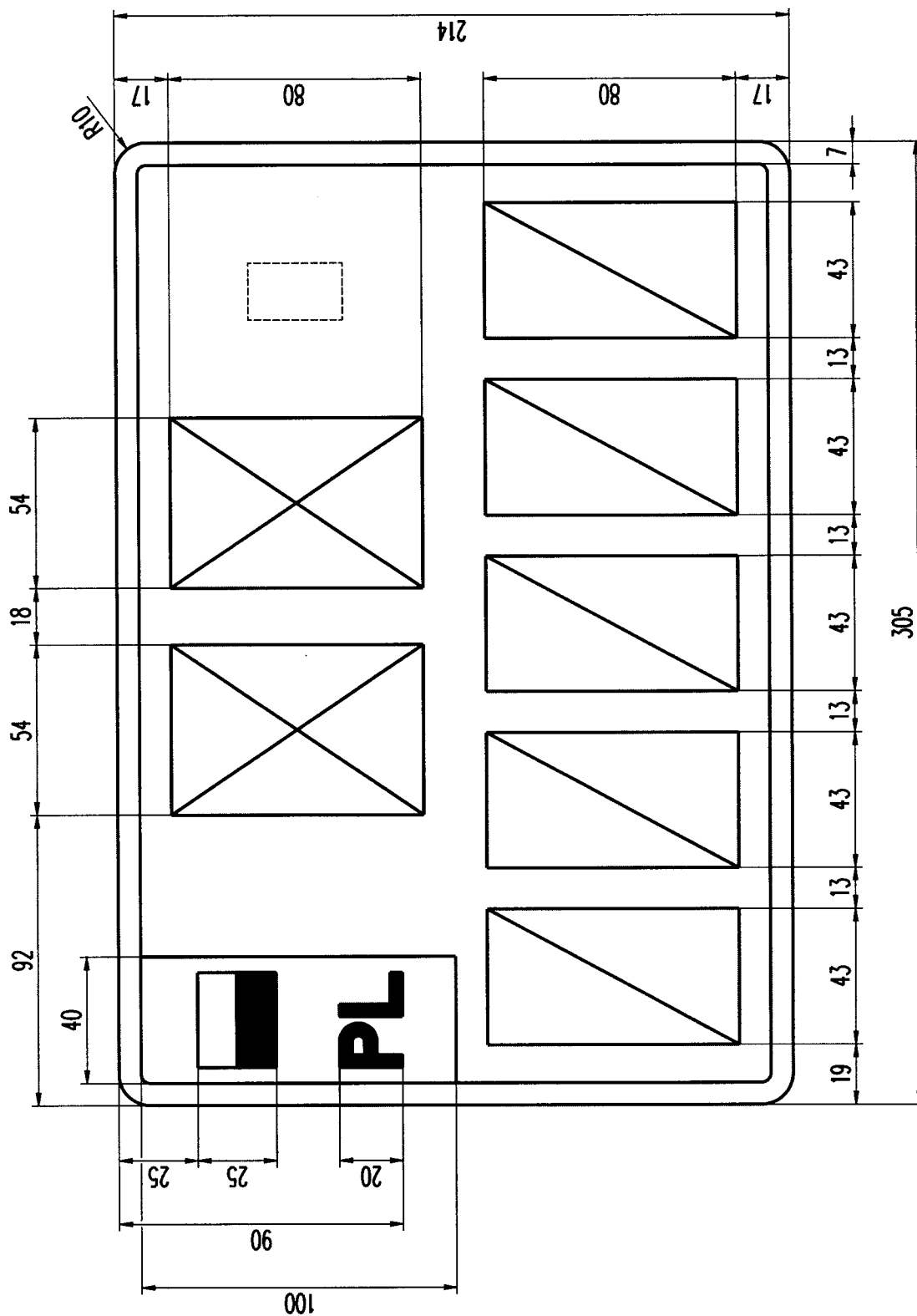
Rysunek 19. Tablica samochodowa zwyczajna dwurzędowa (2 litery, 5 cyfr)
