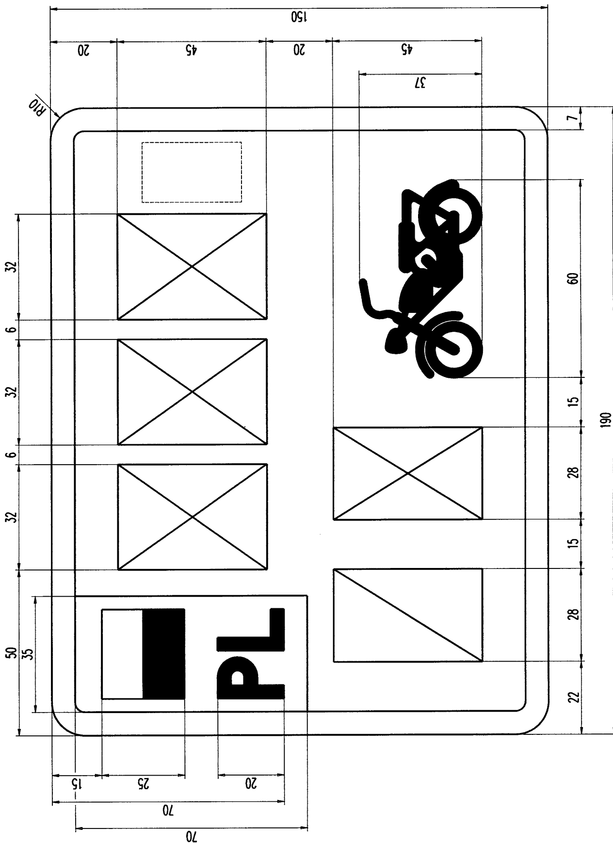
Rysunek 55. Tablica motocyklowa zabytkowa (3 litery, 1 cyfra, 1 litera)
