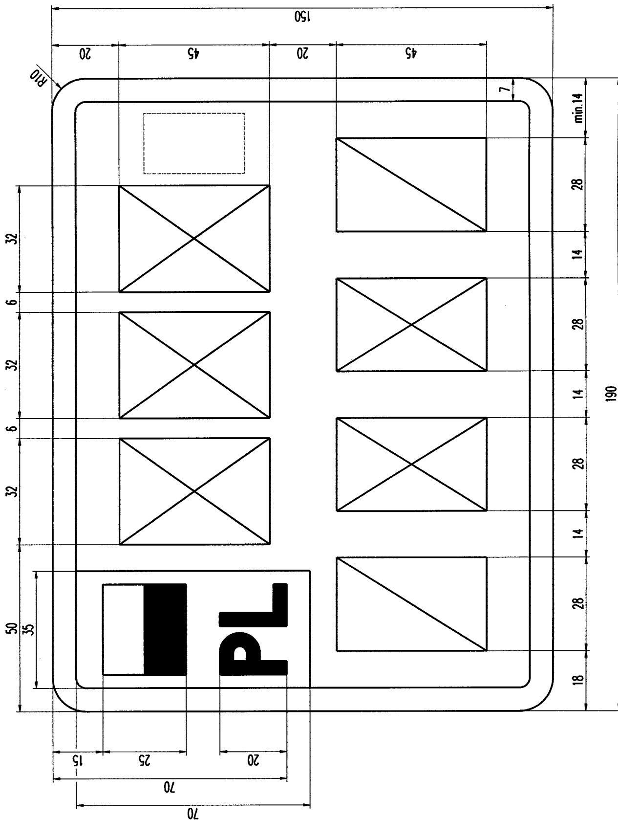
Rysunek 39. Tablica motocyklowa zwyczajna (3 litery, 1 cyfra, 2 litery, 1 cyfra)
