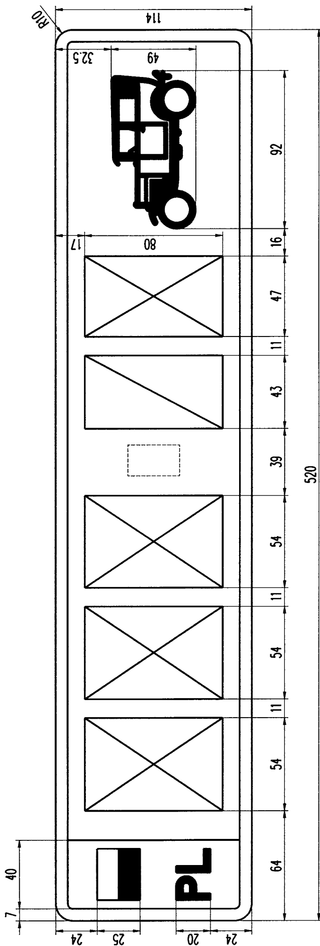
Rysunek 51. Tablica samochodowa zabytkowa jednorzędowa (3 litery, 1 cyfra, 1 litera)
