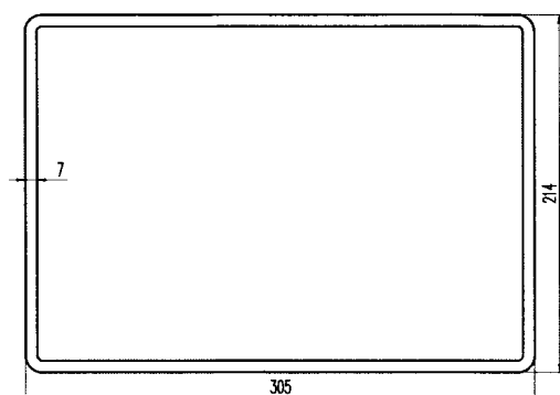
Tablica samochodowa dwurzędowa
