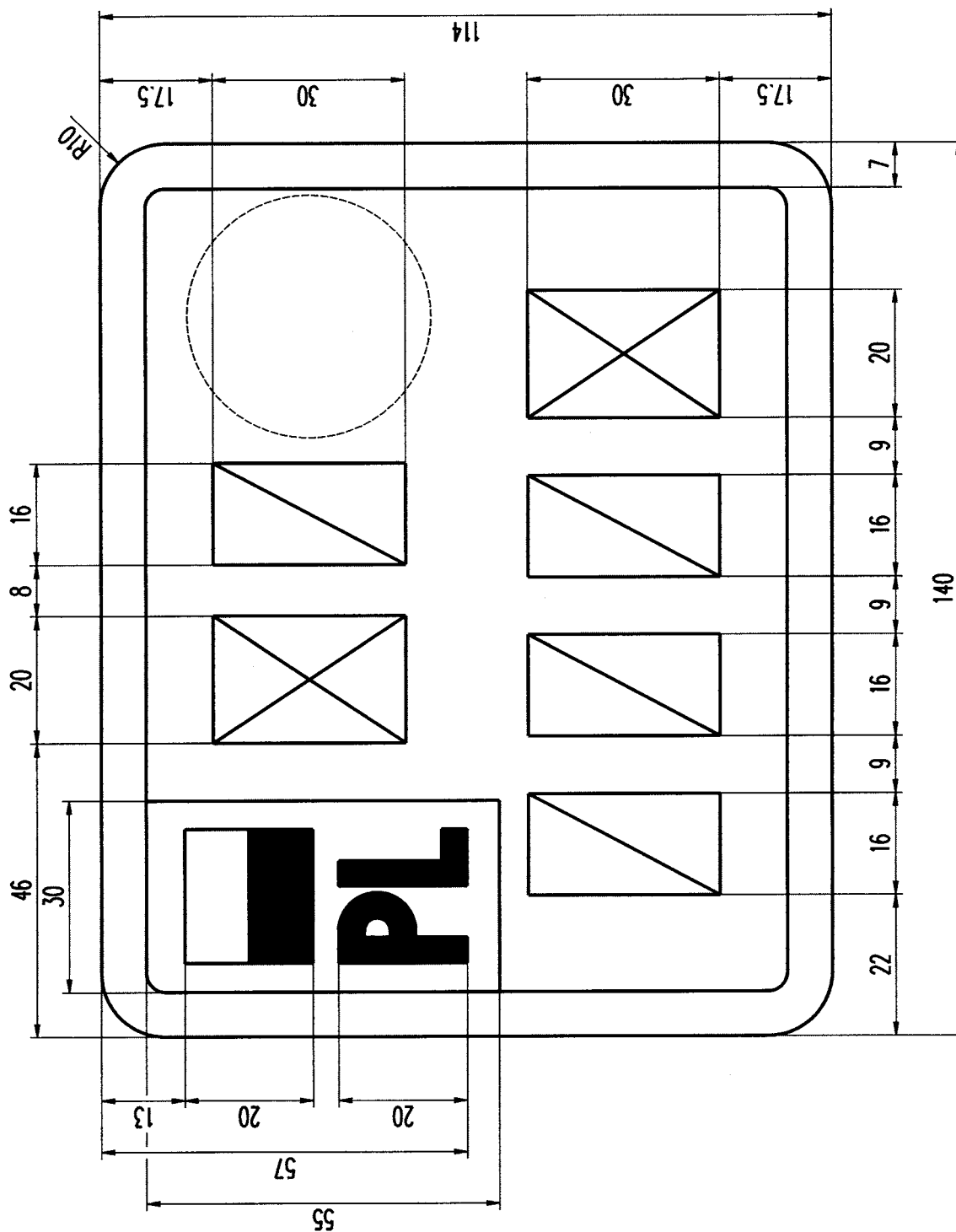
Rysunek 66. Tablica motorowerowa tymczasowa (1 litera, 1 cyfra, 3 cyfry, 1 litera)
