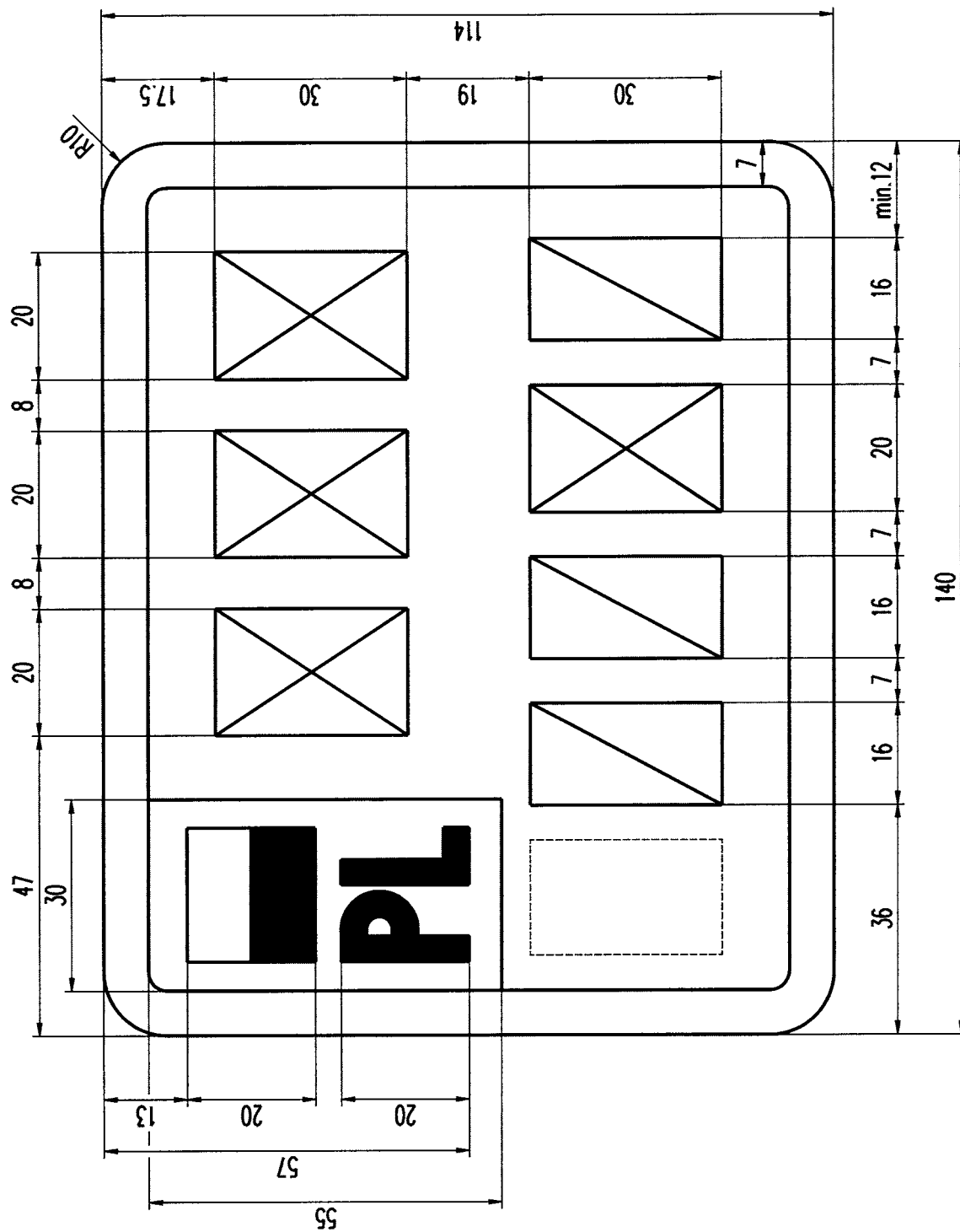
Rysunek 47. Tablica motorowerowa zwyczajna (3 litery, 2 cyfry, 1 litera, 1 cyfra)
