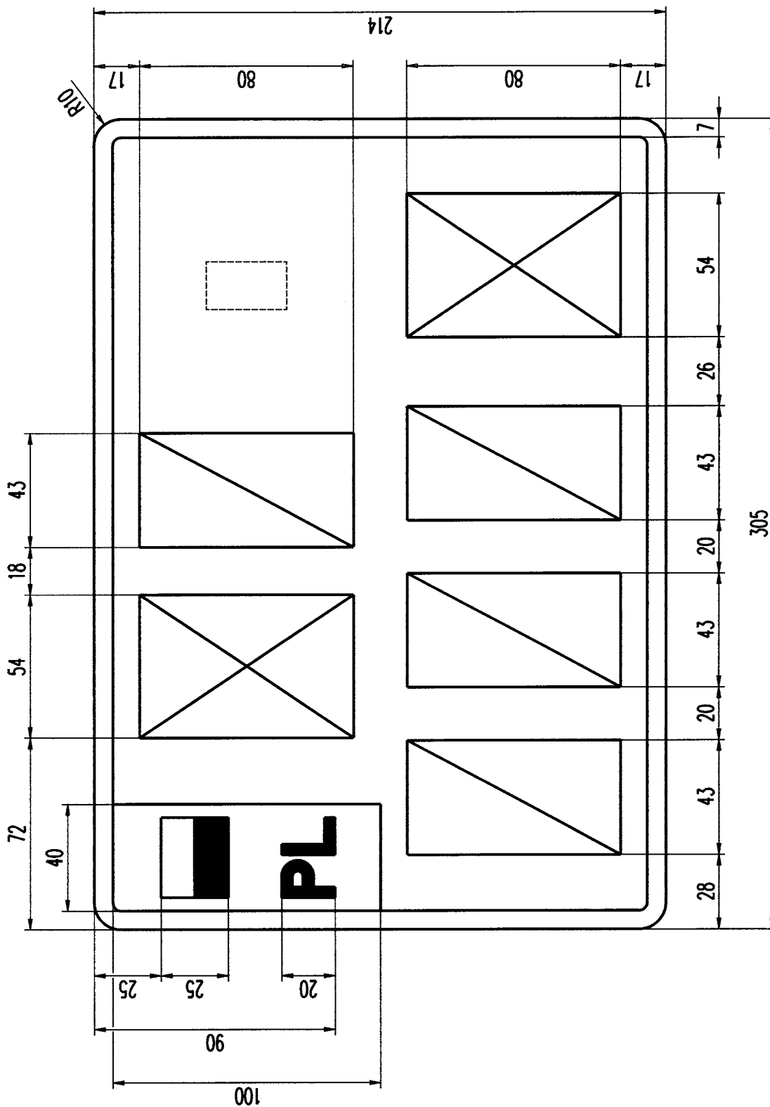
Rysunek 61. Tablica samochodowa tymczasowa dwurzędowa badawcza
