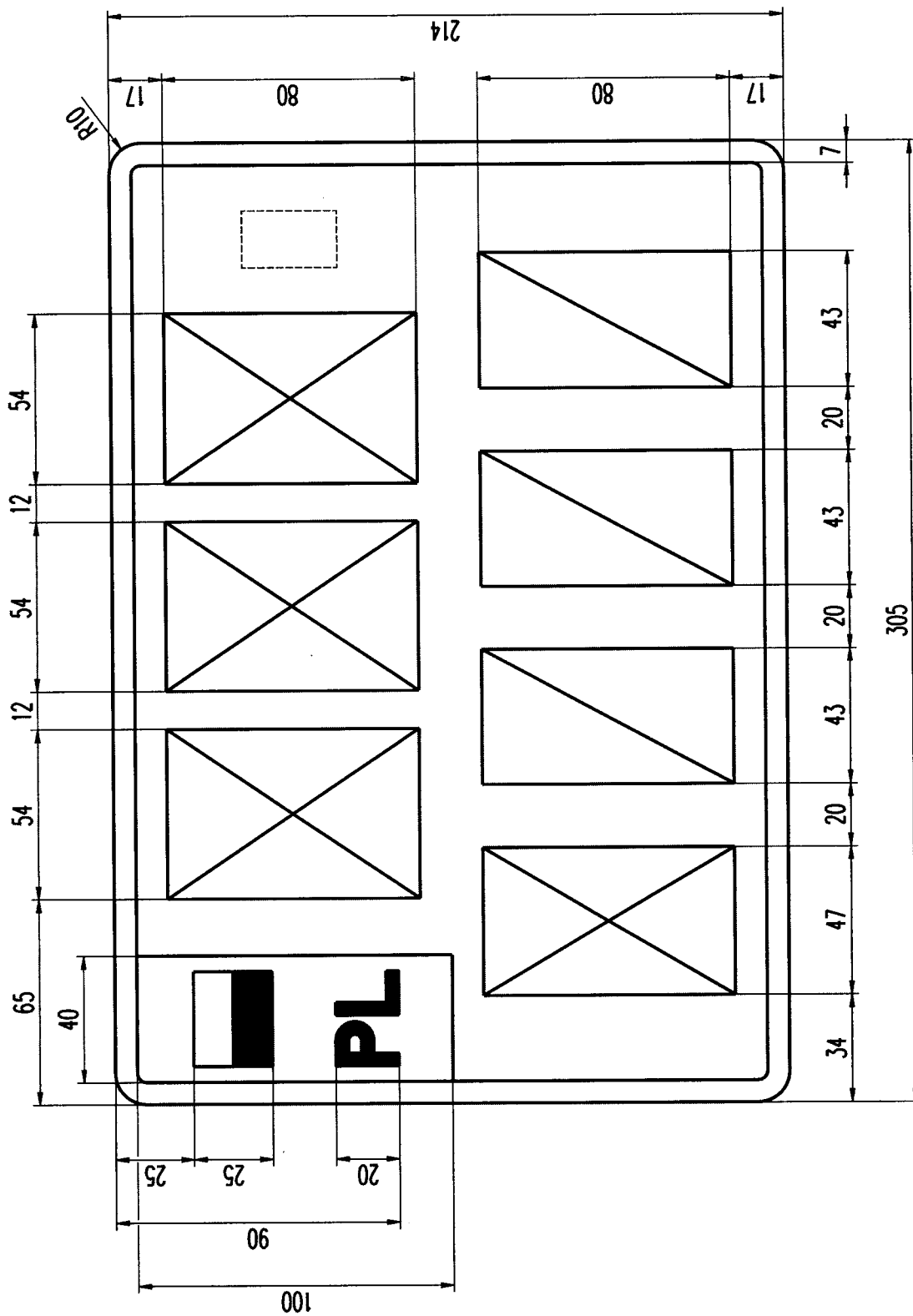
Rysunek 22. Tablica samochodowa zwyczajna dwurzędowa (3 litery, 1 litera, 3 cyfry)
