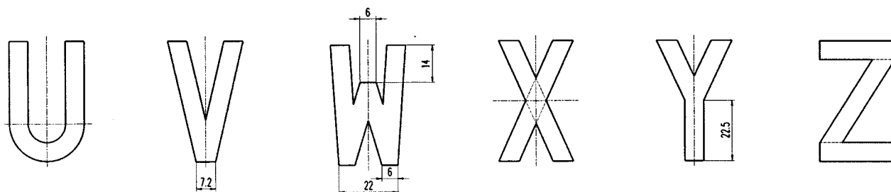
Rysunek 9. Wzory zwężonych liter do tablic motocyklowych
