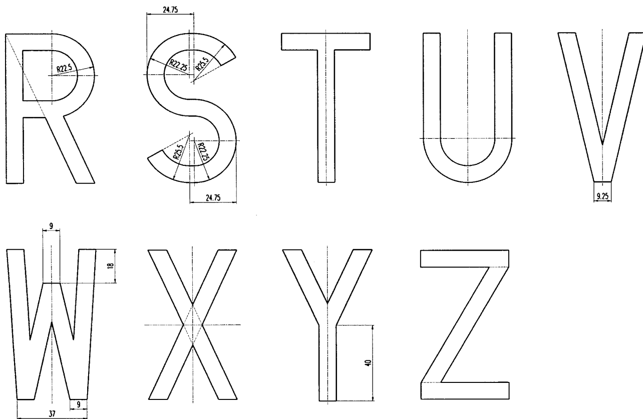
Rysunek 7. Wzory zwężonych liter do tablic samochodowych
