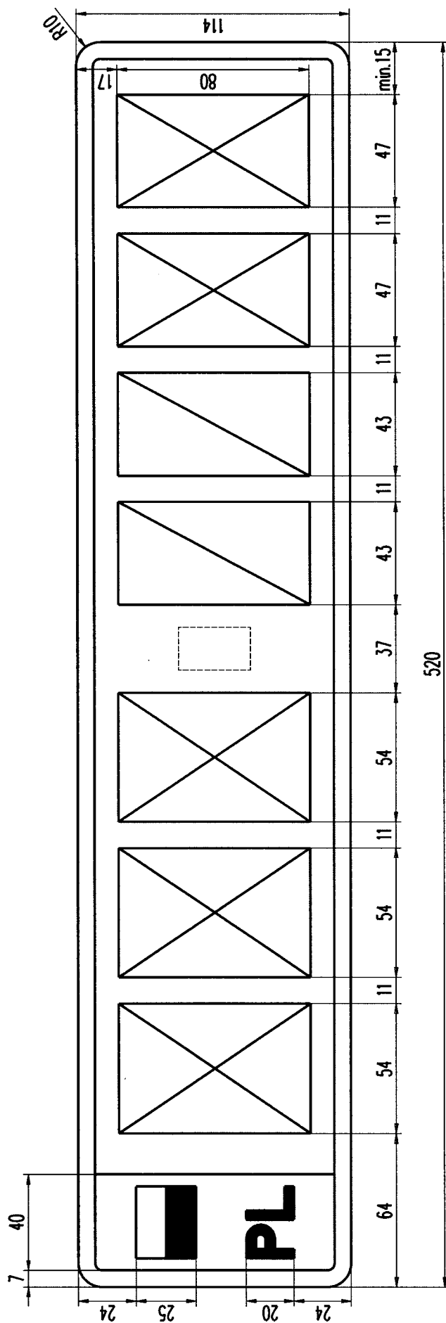
Rysunek 17. Tablica samochodowa zwyczajna jednorzędowa (3 litery, 2 cyfry, 2 litery)
