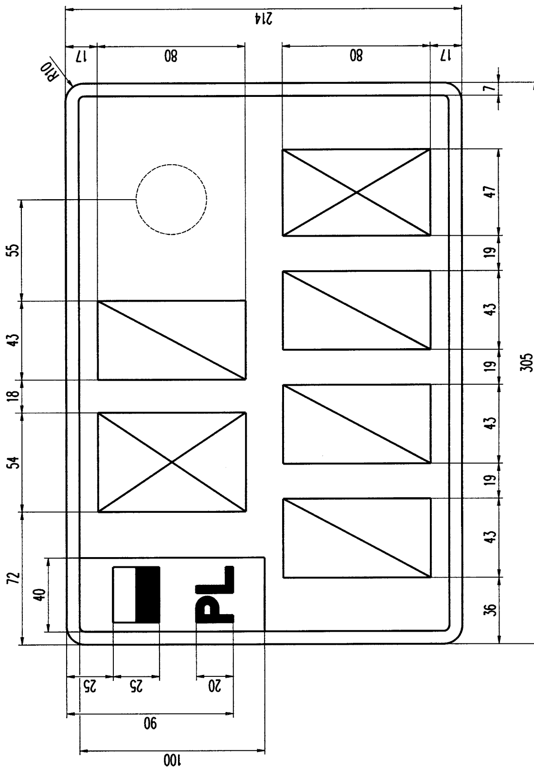
Rysunek 60. Tablica samochodowa tymczasowa dwurzędowa (1 litera, 1 cyfra, 3 cyfry, 1 litera)
