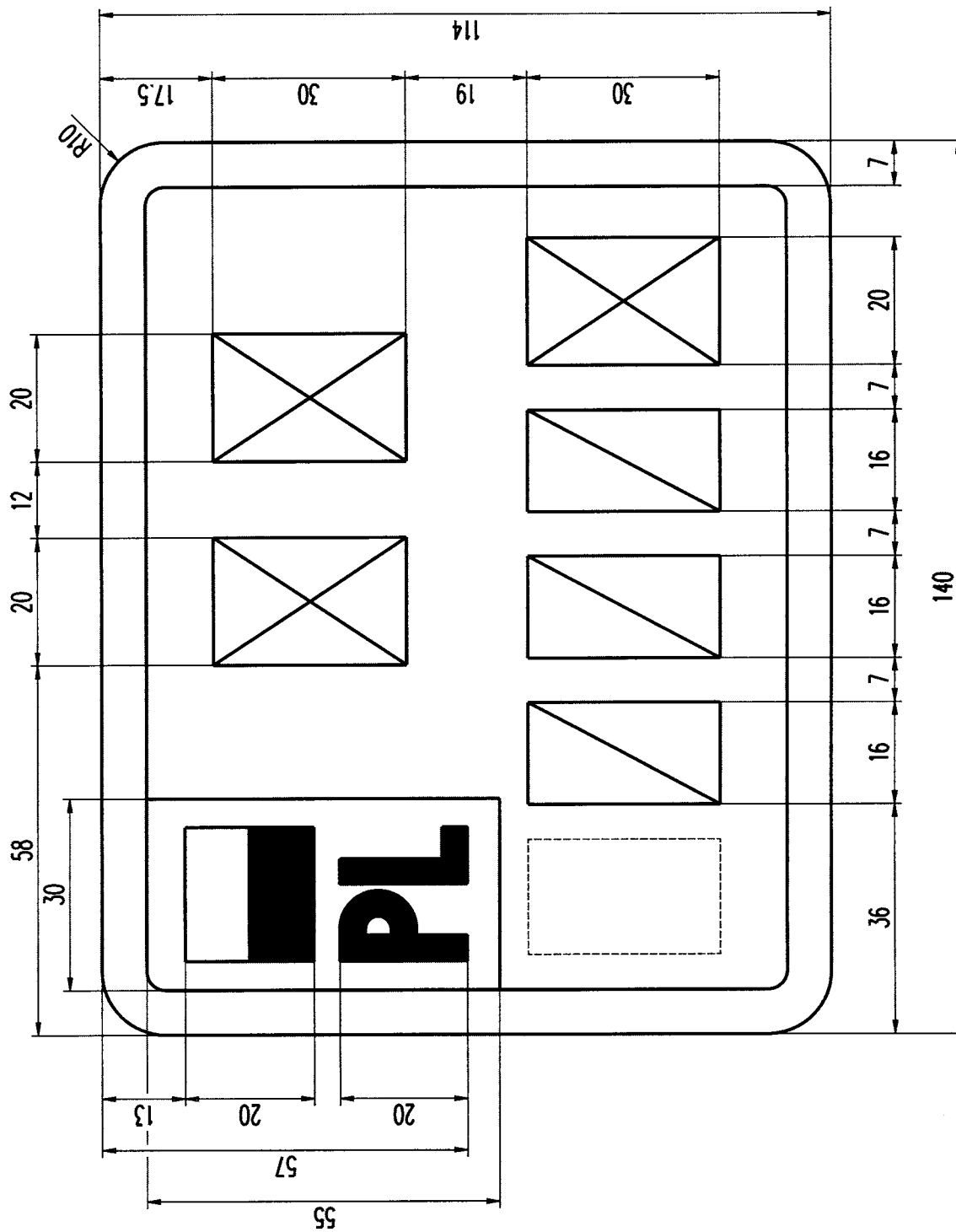
Rysunek 44. Tablica motorowerowa zwyczajna (2 litery, 3 cyfry, 1 litera)
