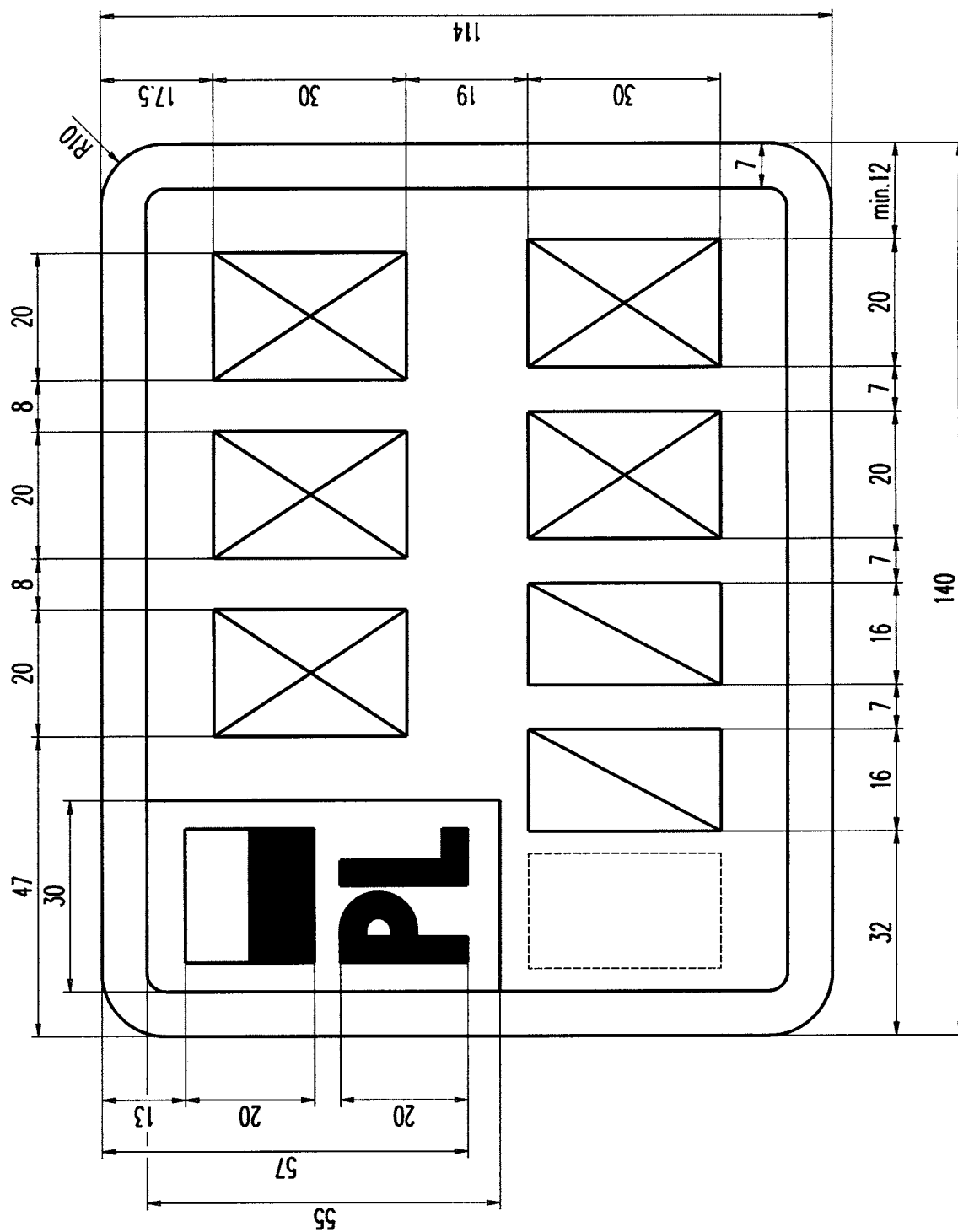
Rysunek 48. Tablica motorowerowa zwyczajna (3 litery, 2 cyfry, 2 litery)
