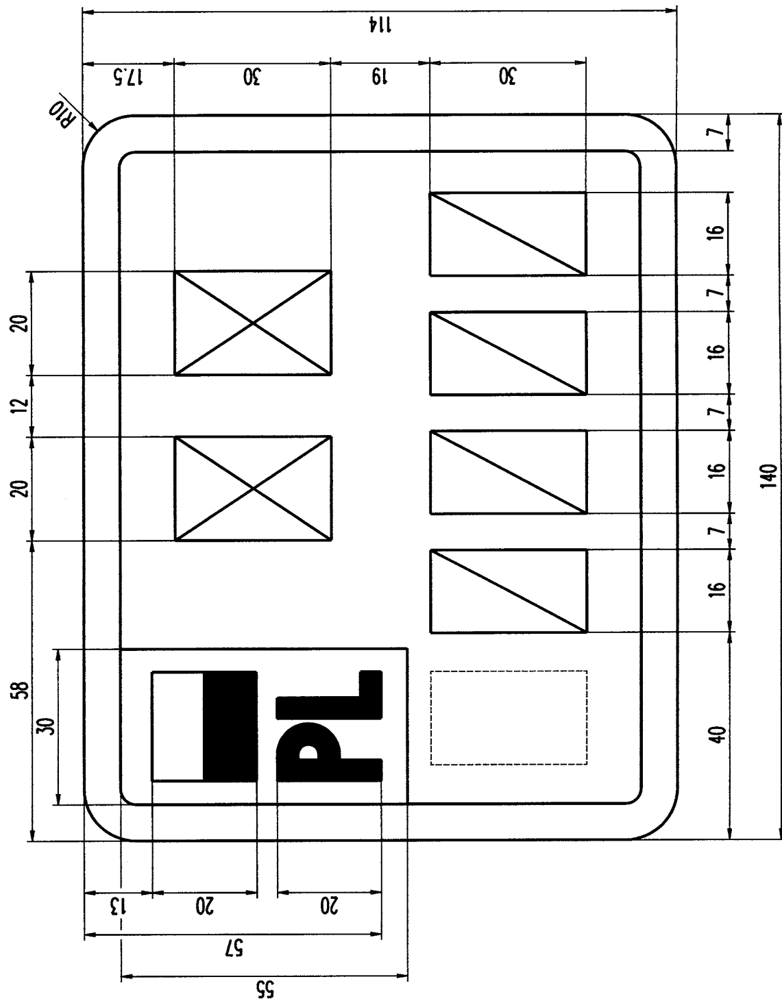
Rysunek 43. Tablica motorowerowa zwyczajna (2 litery, 4 cyfry)
