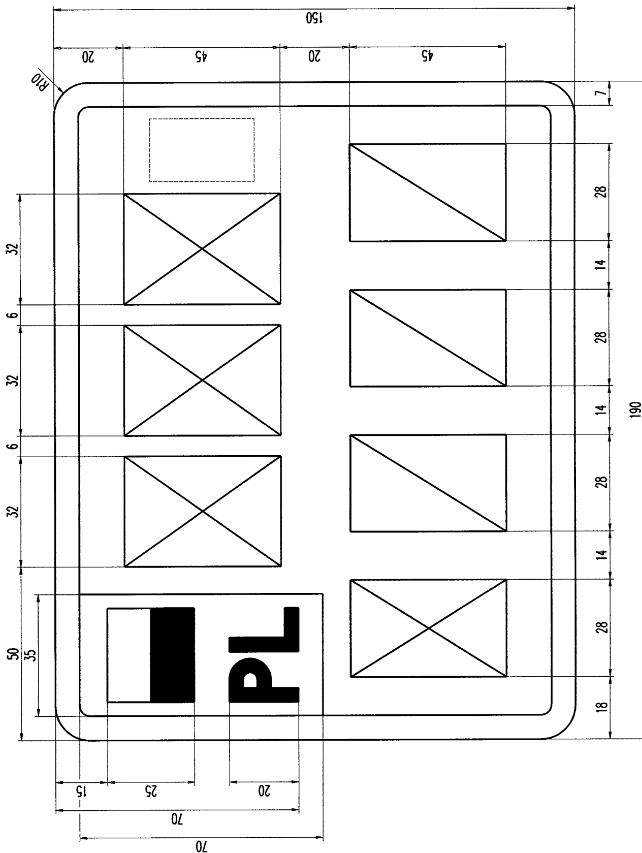
Rysunek 35. Tablica motocyklowa zwyczajna (3 litery, 1 litera, 3 cyfry)
