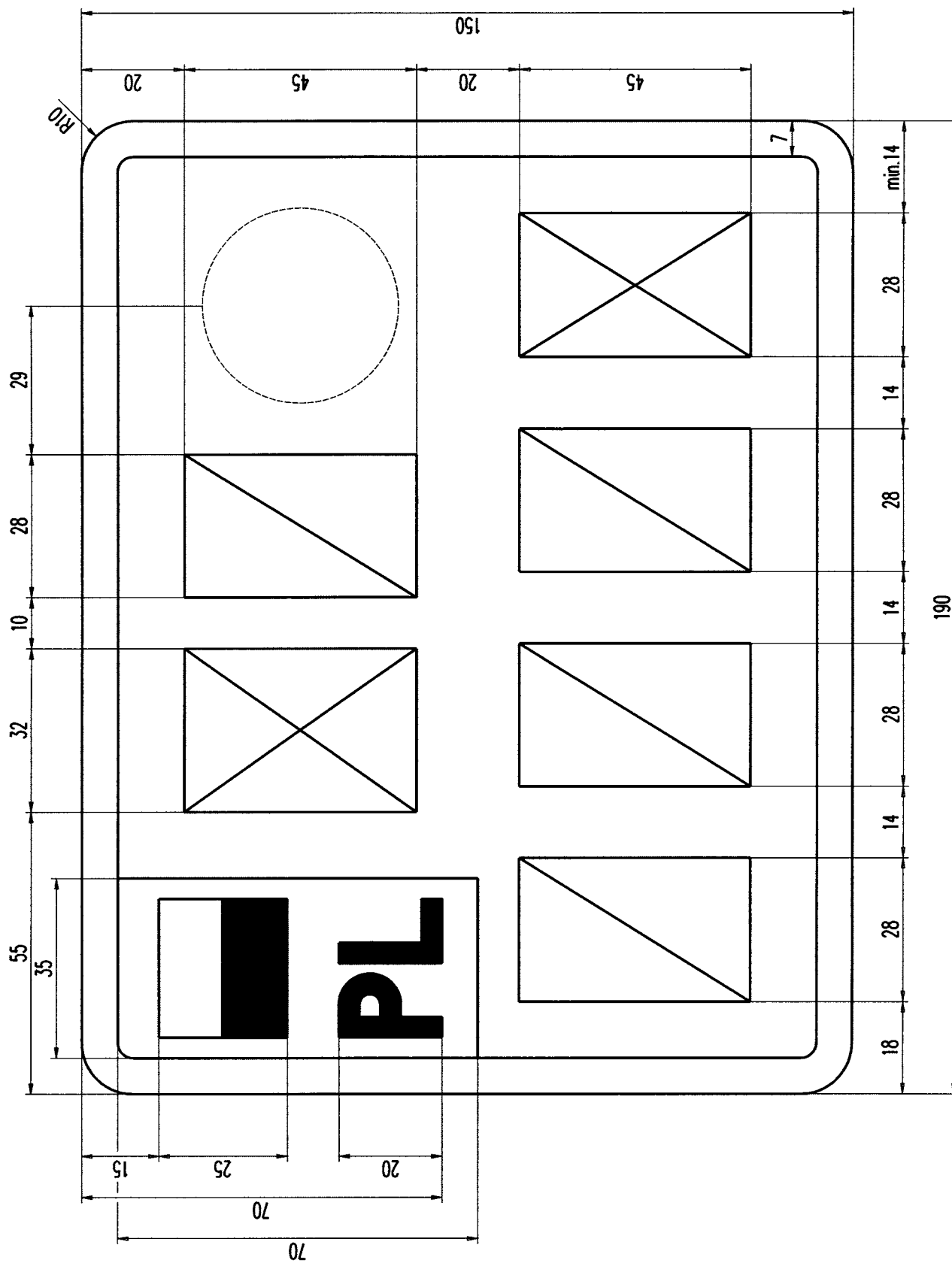
Rysunek 63. Tablica motocyklowa tymczasowa (1 litera, 1 cyfra, 3 cyfry, 1 litera)
