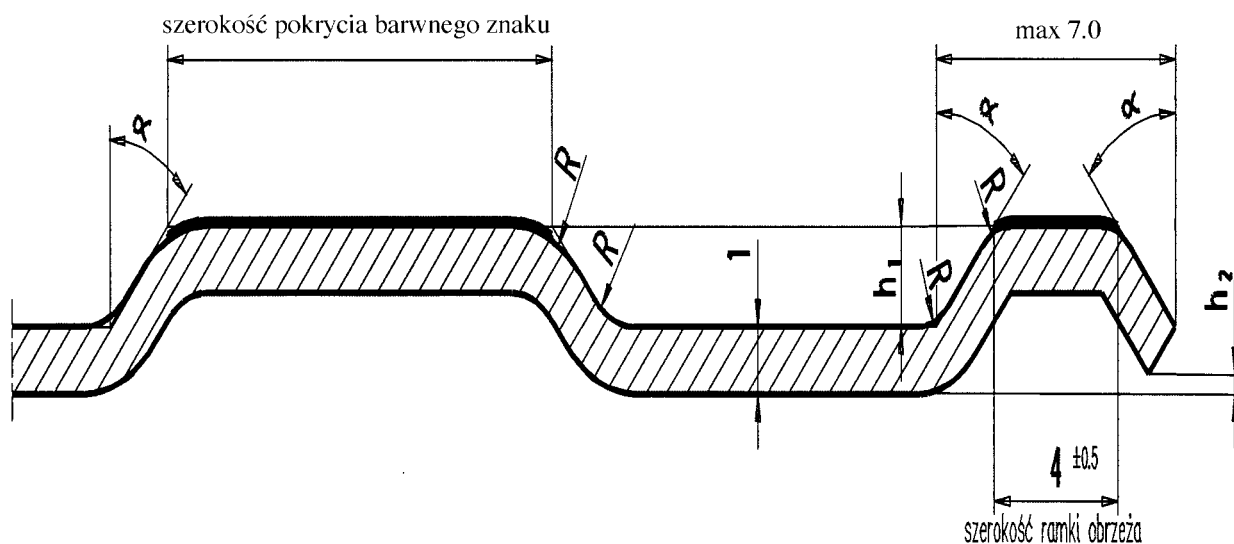
Rysunek 2. Kształt przetłoczeń znaków i ramki obrzeża
