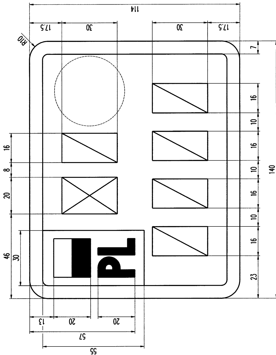
Rysunek 65. Tablica motorowerowa tymczasowa (1 litera, 1 cyfra, 4 cyfry)
