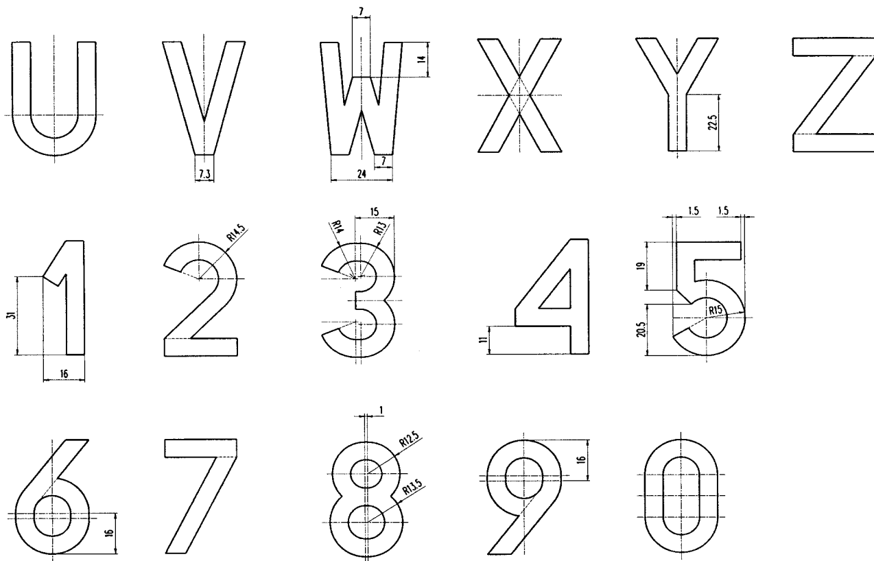
Rysunek 8. Wzory liter i cyfr do tablic motocyklowych
