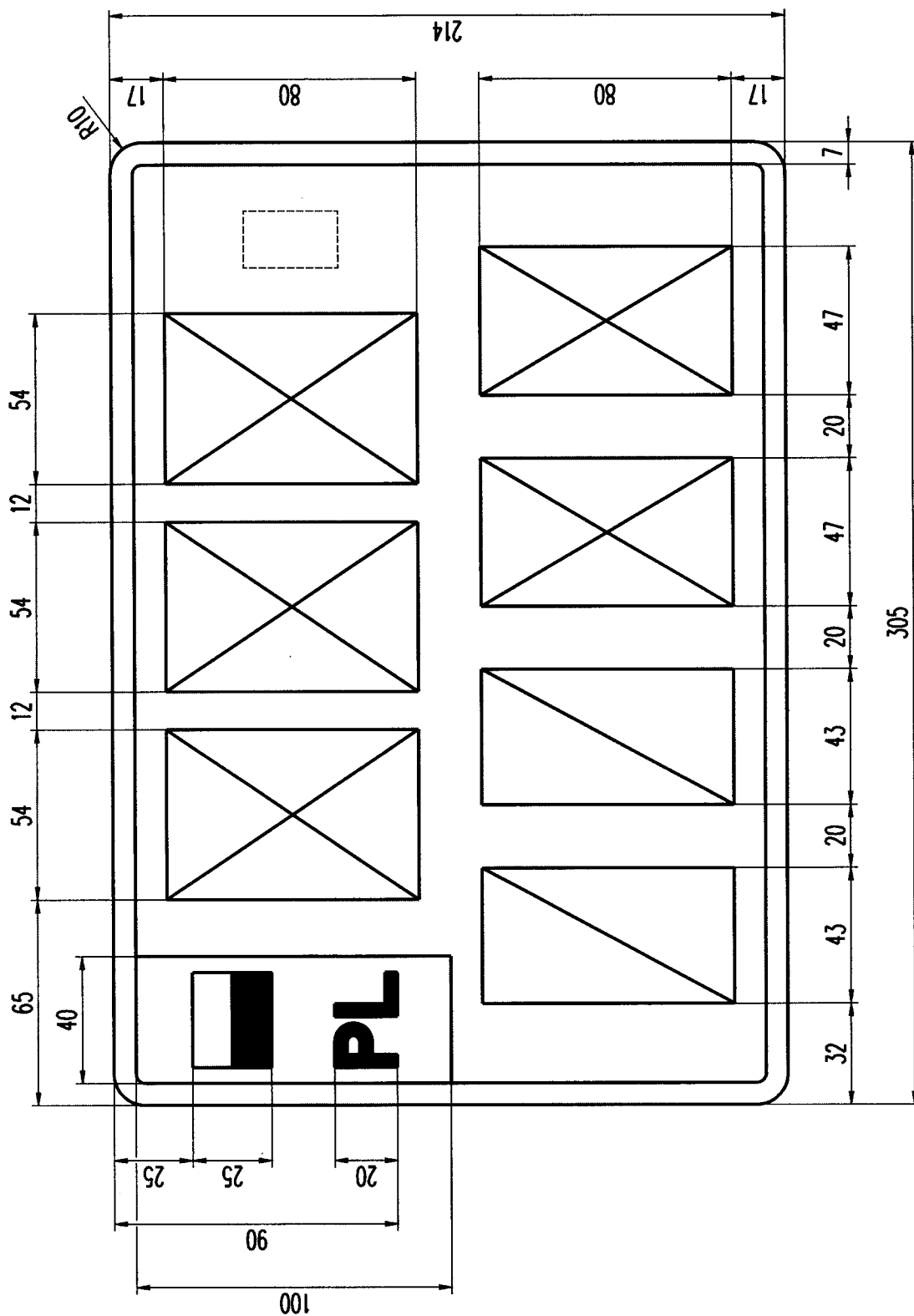
Rysunek 25. Tablica samochodowa zwyczajna dwurzędowa (3 litery, 2 cyfry, 2 litery)
