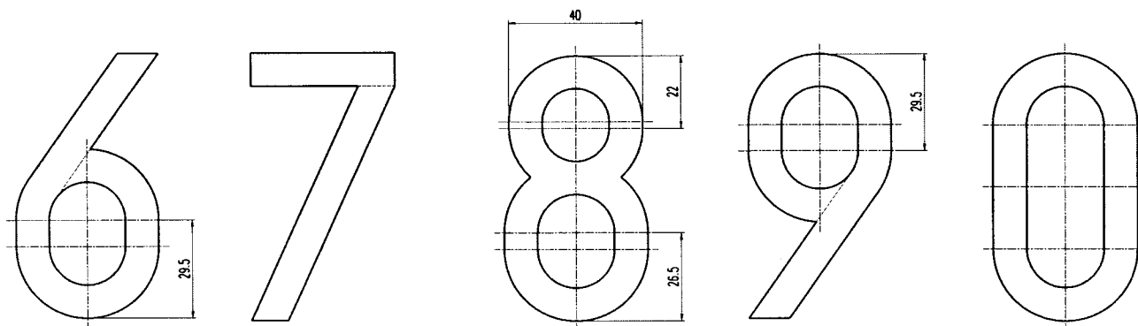
Rysunek 6. Wzory liter i cyfr do tablic samochodowych
