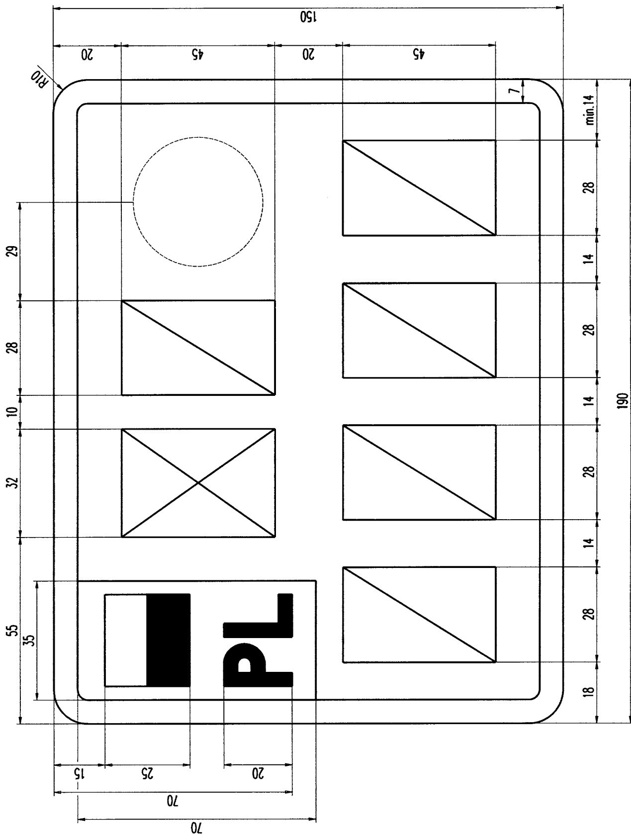
Rysunek 62. Tablica motocyklowa tymczasowa (1 litera, 1 cyfra, 4 cyfry)
