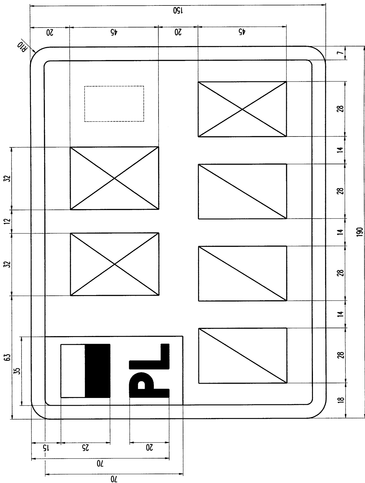
Rysunek 34. Tablica motocyklowa zwyczajna (2 litery, 3 cyfry, 1 litera)
