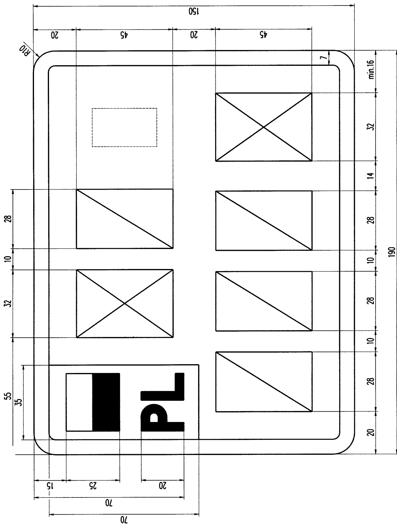
Rysunek 64. Tablica motocyklowa tymczasowa badawcza
