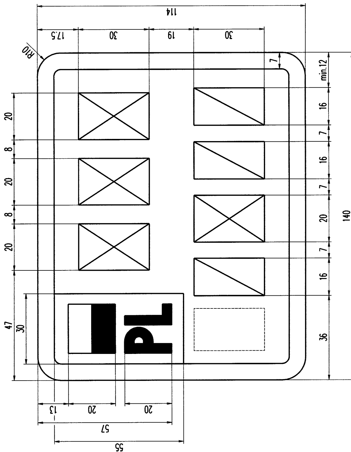
Rysunek 46. Tablica motorowerowa zwyczajna (3 litery, 1 cyfra, 1 litera, 2 cyfry)
