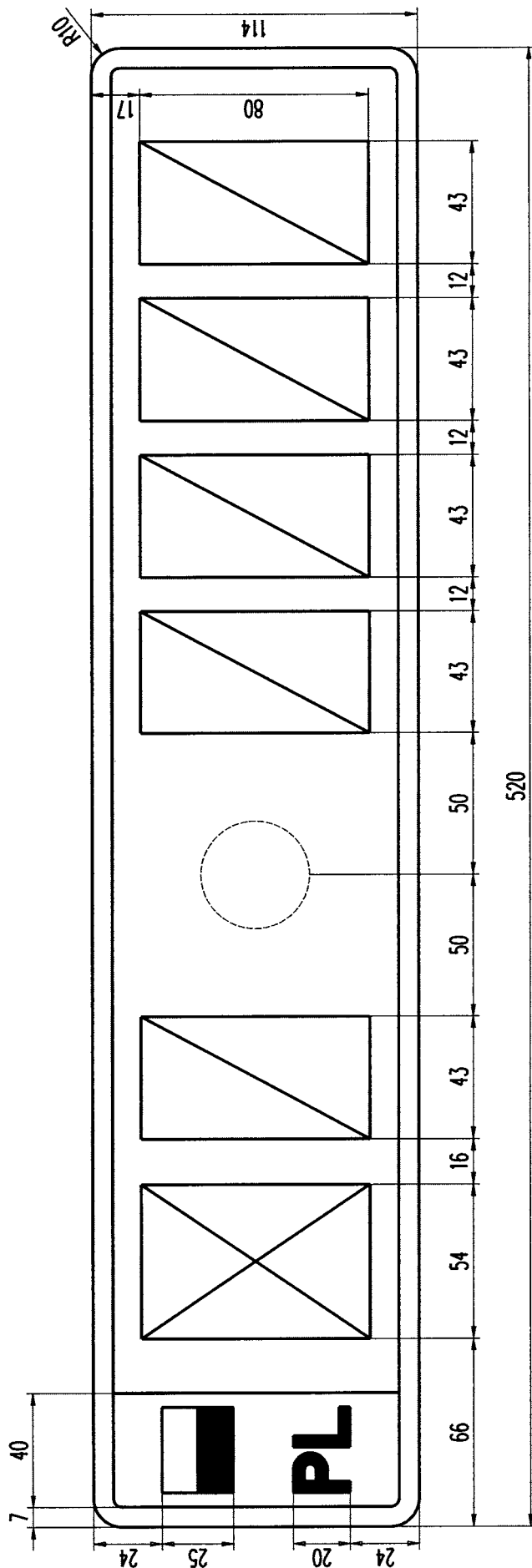
Rysunek 56. Tablica samochodowa tymczasowa jednorzędowa (1 litera, 1 cyfra, 4 cyfry)
