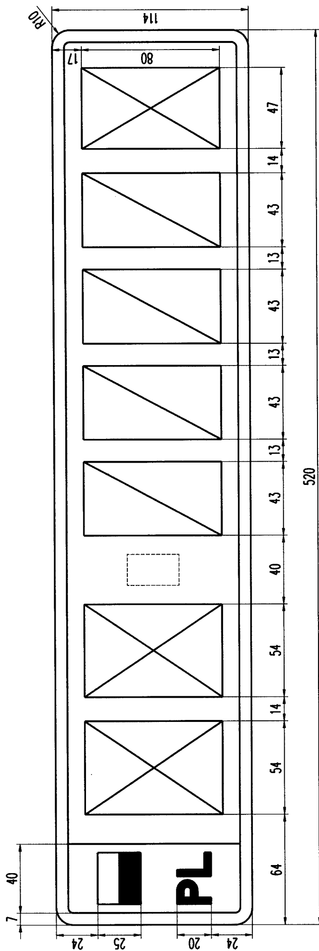
Rysunek 12. Tablica samochodowa zwyczajna jednorzędowa (2 litery, 4 cyfry, 1 litera)
