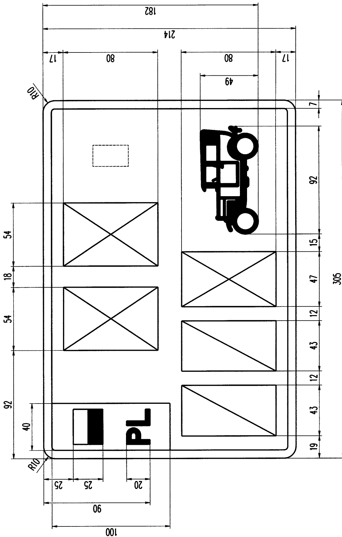
Rysunek 52. Tablica samochodowa zabytkowa dwurzędowa (2 litery, 2 cyfry, 1 litera)
