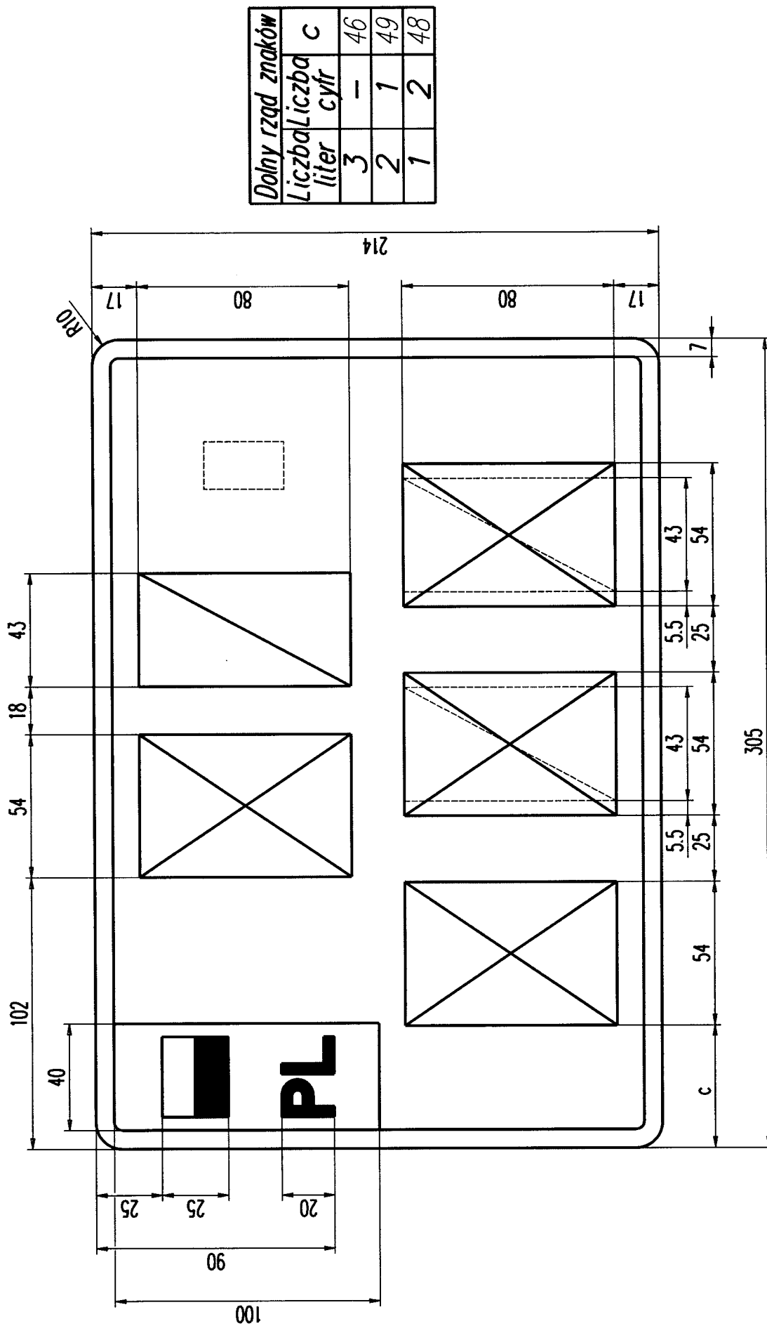
Rysunek 32. Tablica samochodowa indywidualna dwurzędowa
