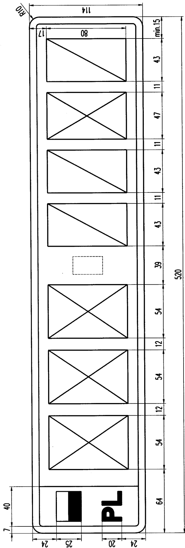
Rysunek 16. Tablica samochodowa zwyczajna jednorzędowa (3 litery, 2 cyfry, 1 litera, 1 cyfra)
