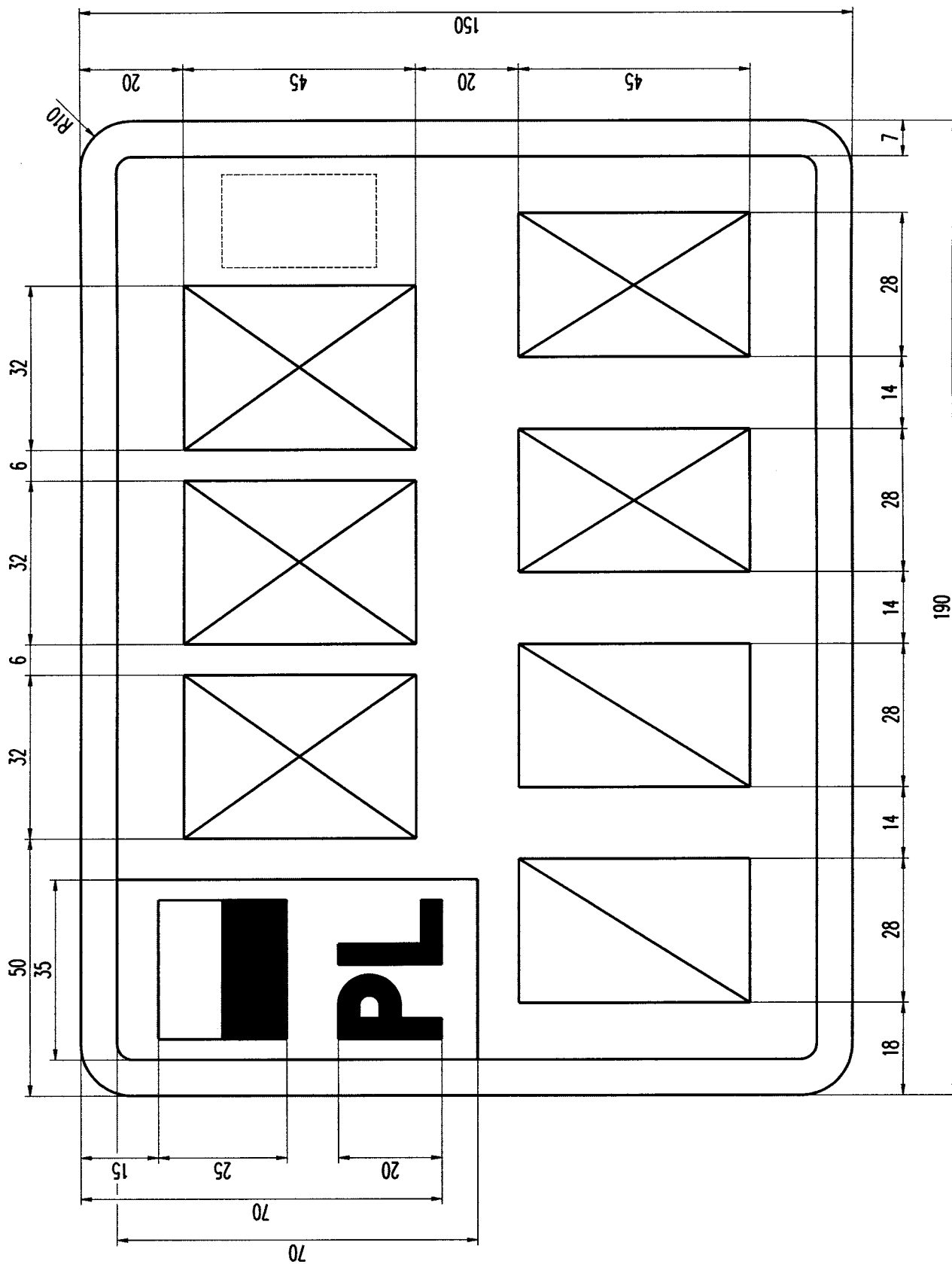
Rysunek 38. Tablica motocyklowa zwyczajna (3 litery, 2 cyfry, 2 litery)
