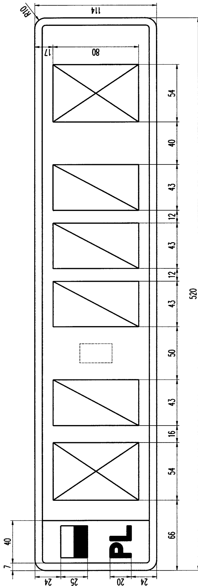
Rysunek 58. Tablica samochodowa tymczasowa jednorzędowa badawcza
