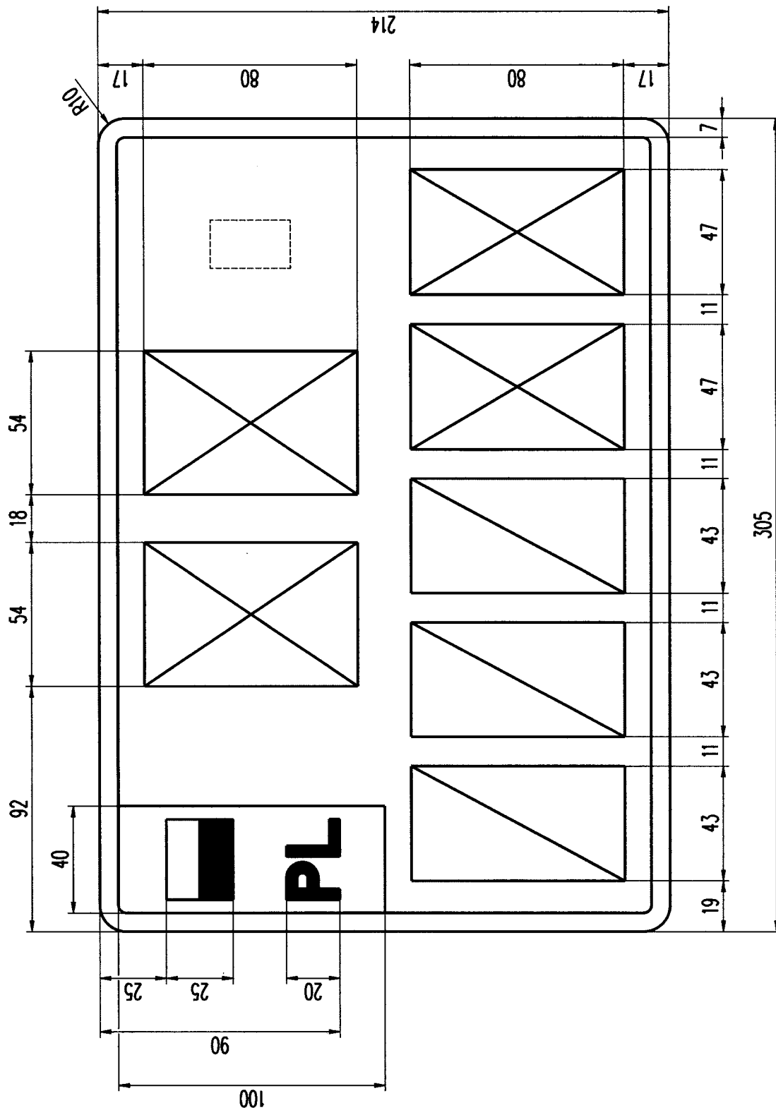
Rysunek 21. Tablica samochodowa zwyczajna dwurzędowa (2 litery, 3 cyfry, 2 litery)
