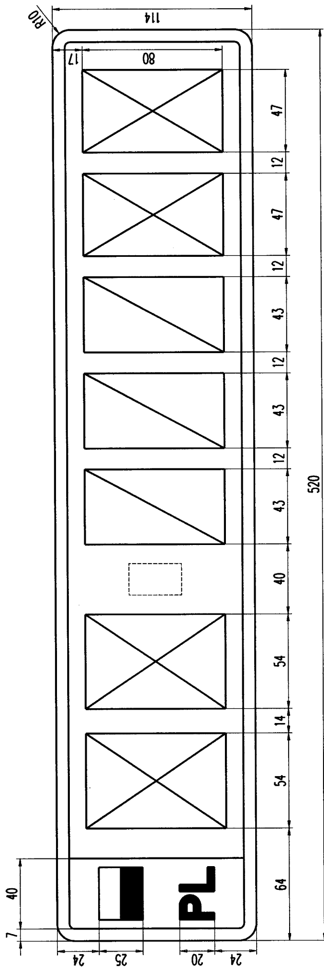
Rysunek 13. Tablica samochodowa zwyczajna jednorzędowa (2 litery, 3 cyfry, 2 litery)
