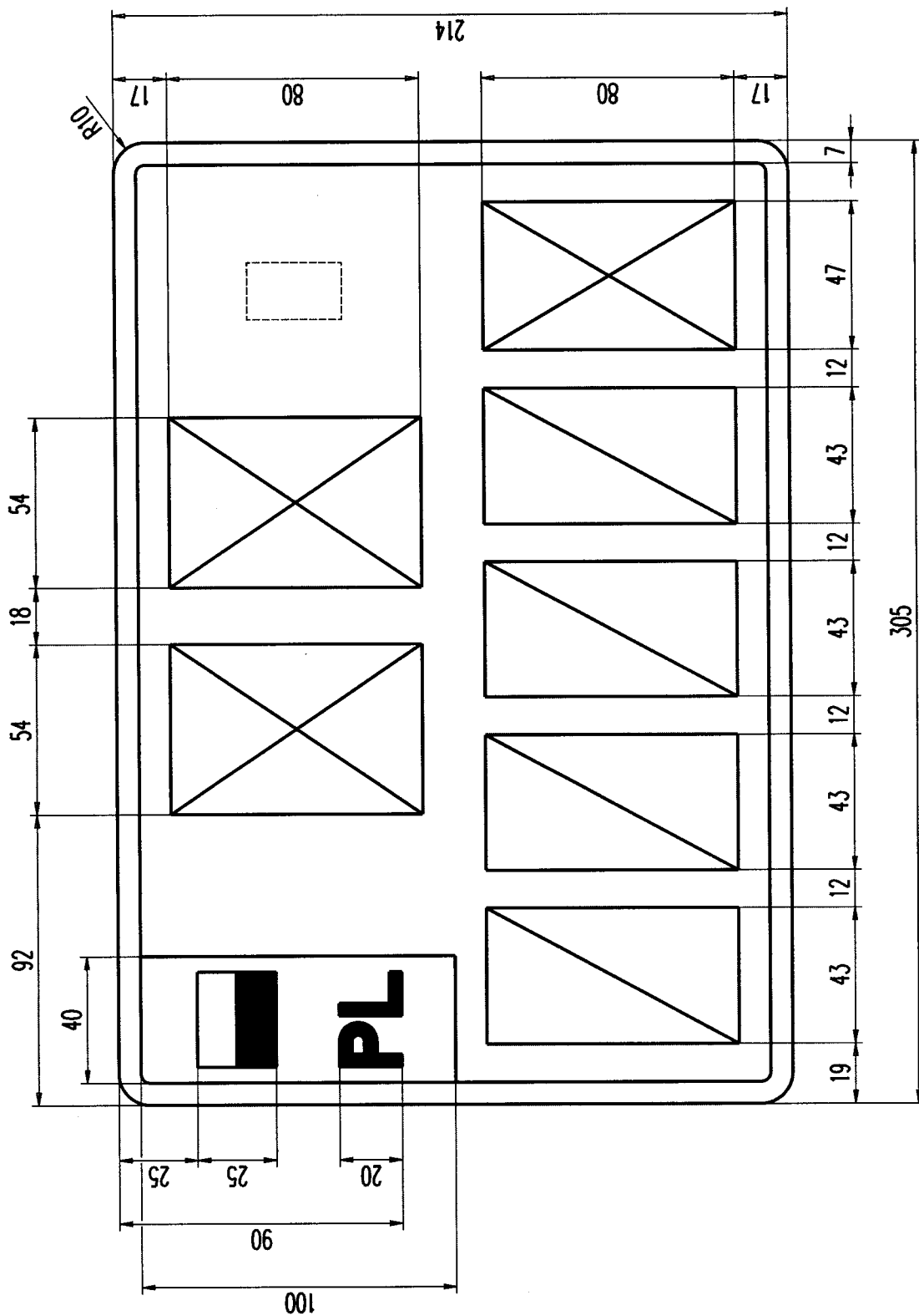
Rysunek 20. Tablica samochodowa zwyczajna dwurzędowa (2 litery, 4 cyfry, 1 litera)
